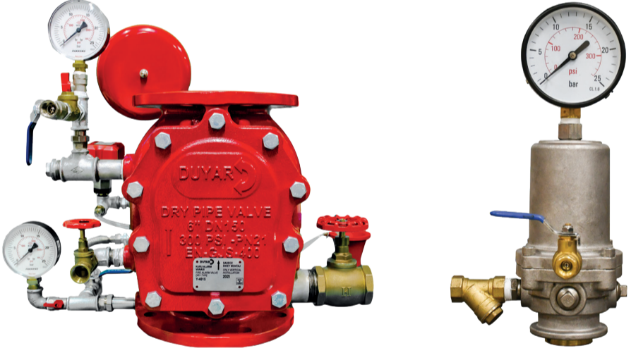
KURU ALARM VANASI ve HIZLANDIRICISI Y-4015 | Y-4016
